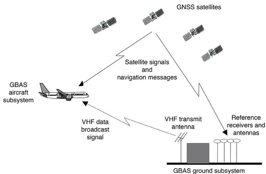
Figura 3.11: Principio operativo de GBAS [Fig14].
