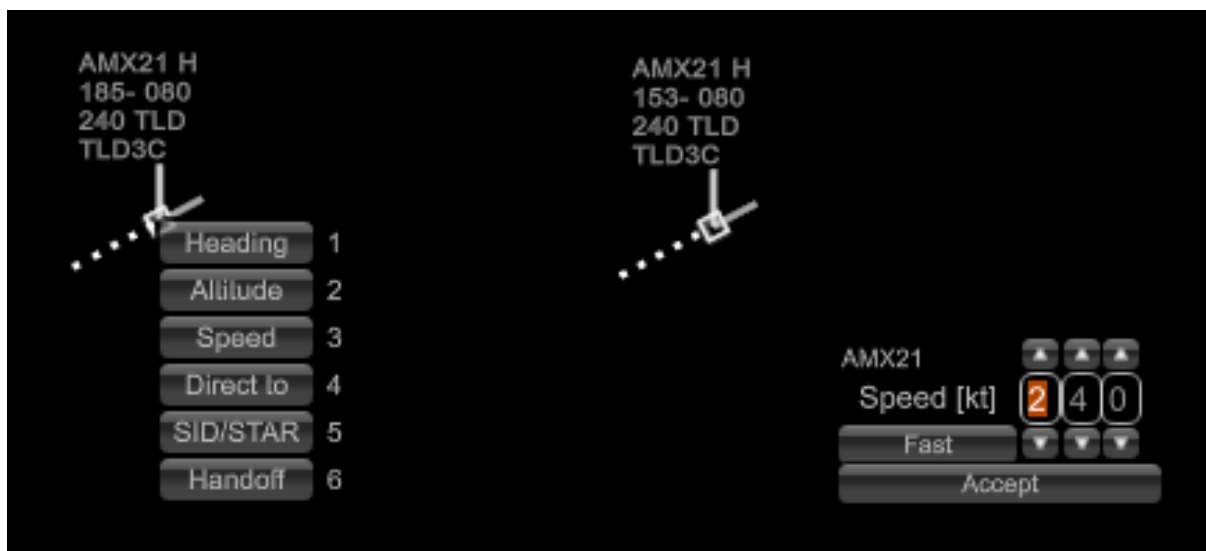
Menú de control ATC y submenú para instruir velocidad ( speed ).
