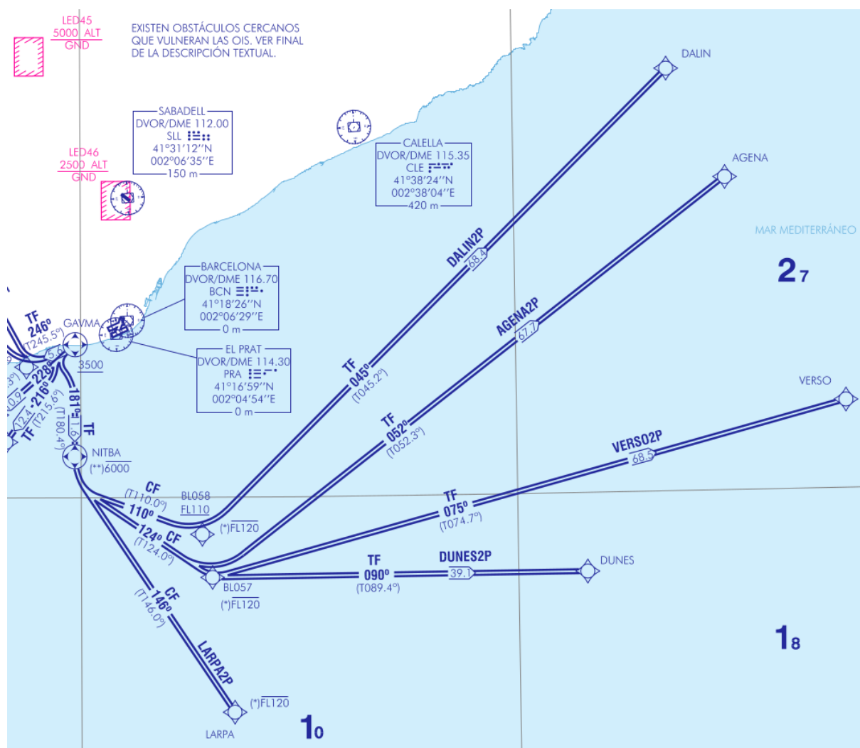
Figura 3.25: Extracto de SID P-RNAV de la RWY 25R de LEBL [Fig30].
