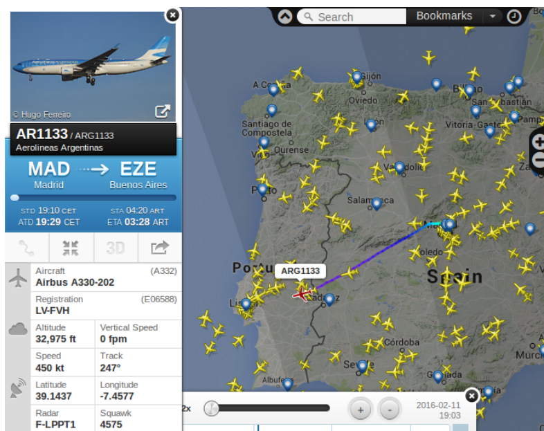
Figura 3.15: Datos ADS-B recogidos por la plataforma Flightradar24 [Fig18].
