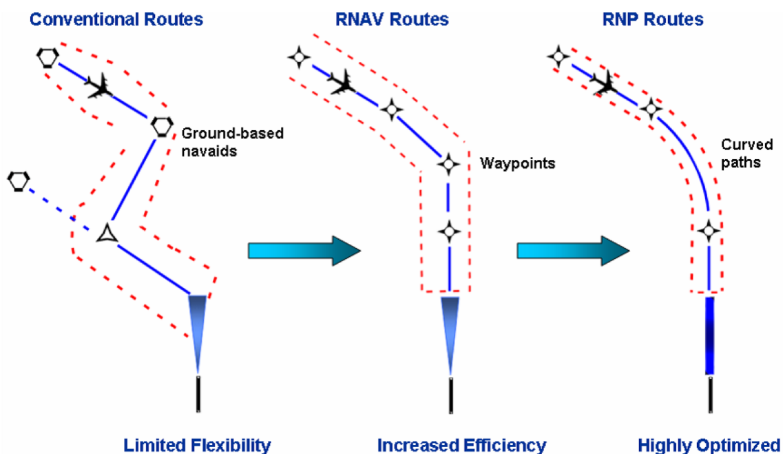
Figura 3.8: Rutas convencionales, RNAV y RNP [Fig12].
